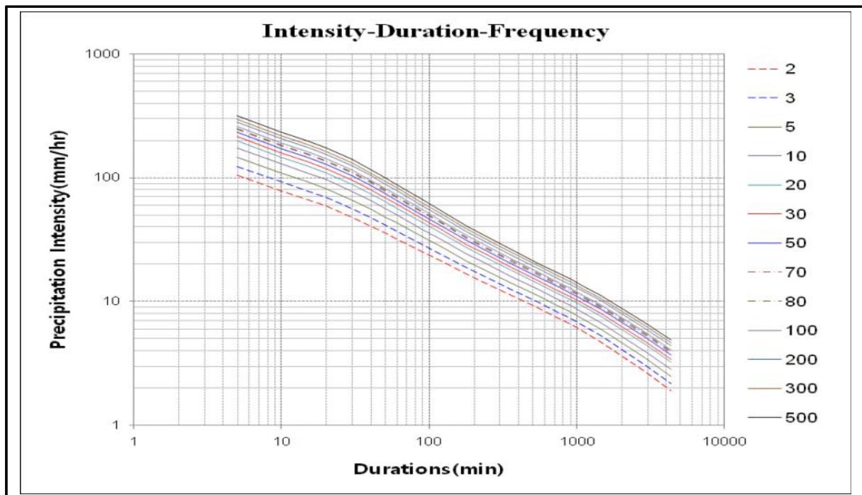
【그림 21.9】 균위지역 IDF곡선
