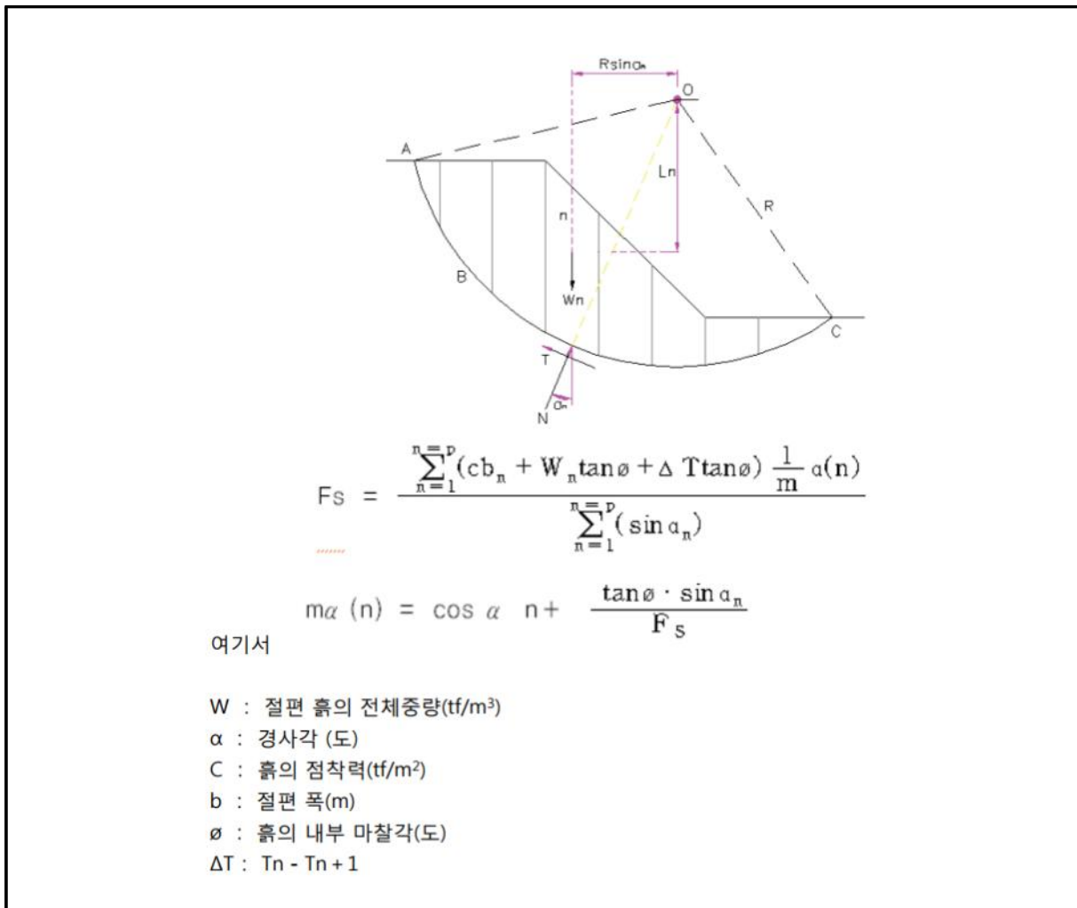
【그림 21.7】 Bishop의 안전율 계산식
